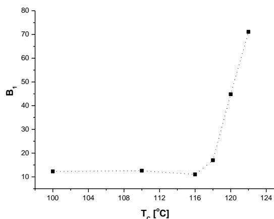
Rys. 2 Zależność współczynnika B_1 od temperatury krystalizacji izotermicznej.
